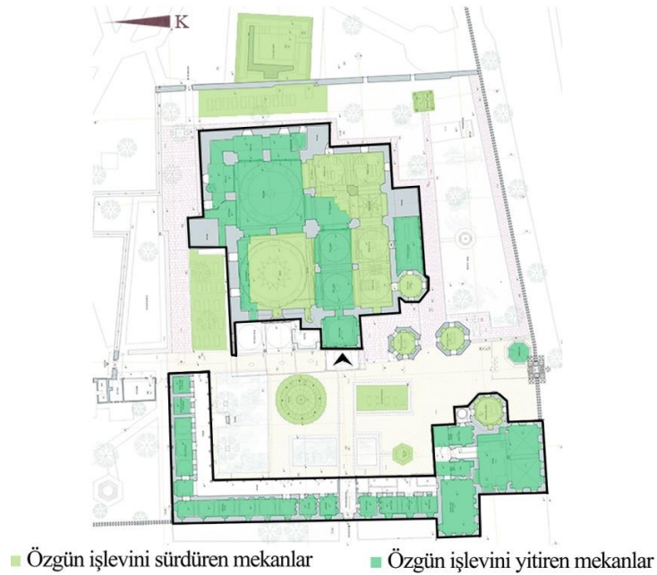
Görsel 4.1.5. Mevlana Dergahı 'nda yer alan mekanların işlev değişikliği durumu (Çizim: Argun Dağıstanlı, 2008; İşlev analizi: Fikret Bademci)
