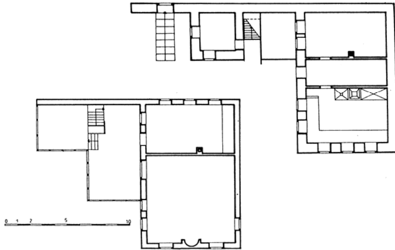
Çizim1: Sareyevo İsa Bey Mevlâhânesi planı (Ayverdi'den).
